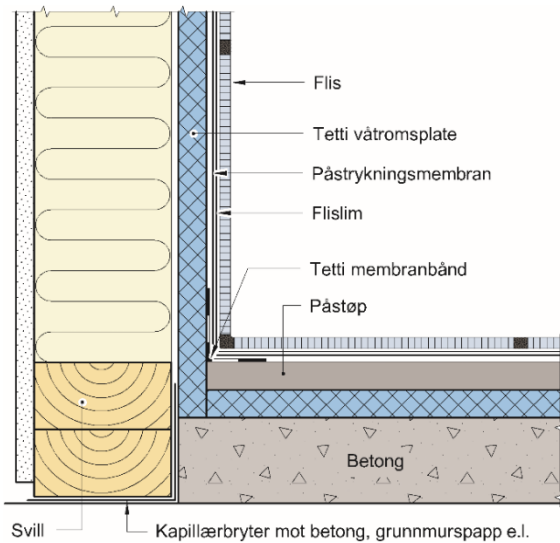
Fig. 4 Eksempel på overgang mellom flisleddt gulv og vegg
