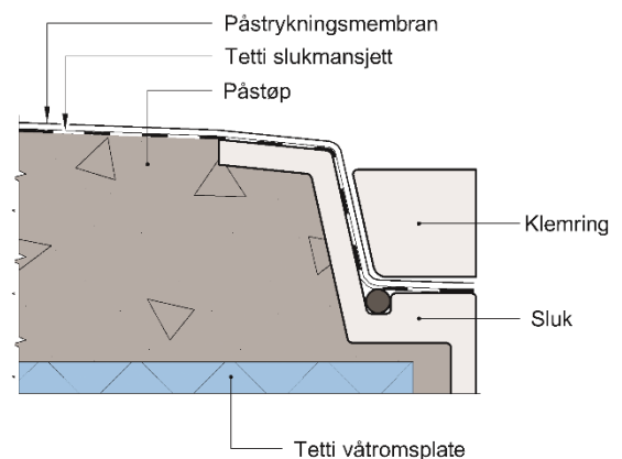
Fig. 6 Eksempel på oppbygging av sluk med klemring
