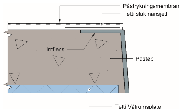
Fig. 7 Eksempel på oppbygging av sluk med limflens
